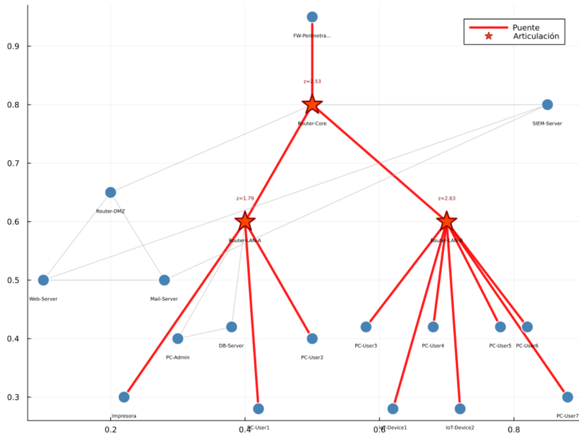
Resiliencia: Nodos de Articulación y Puentes
