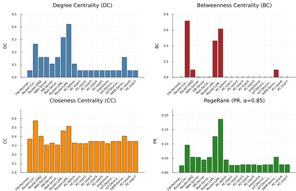
Métricas de Centralidad — Red Corporativa 20 nodos
