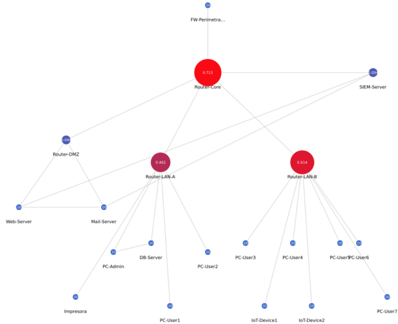
Métricas de Centralidad — Red Corporativa 20 nodos
